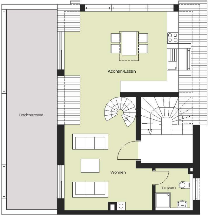
Dachgeschoss
